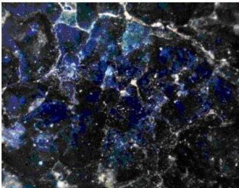
Sapphire bedrock
